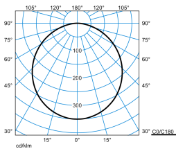
Olisq RWD2 DW 14-40/4/ML-830 PC ET + Olisq RWD2 ZVF 05 (stage 1)
