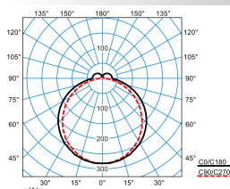
Olisq LWD2 DW 60-8TW ETDD8 IK (DWW)
