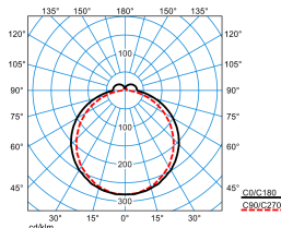
Olisq LWD2 DW 60-8TW ETDD8 IK (DCW)
