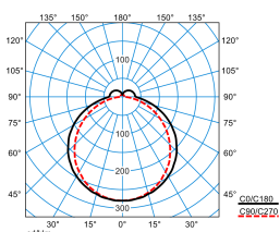
Olisq LWD3 DW 30-8TW ETDD8 IP54 (DCW)
