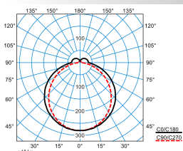
Olisq LWD3 DW 30-8TW ETDD8 IP54 (DWW)
