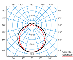
Olisq LWD3 DW 30-8TW ETDD8 IP54 (DSU)
