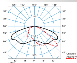
LnPlus 40-AB7L/13500-740 12G1 ETDD (CLO initial value)
