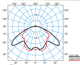
9811IS-LR/2200-840 ET
