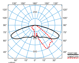
Publisca P1-AB2L-LR/4600-740 6G1S
