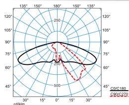
Publisca P1-AB2L-LR/4600-740 6G1S ET (CLO initial value)
