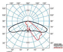
Publisca P1-AB2L-LR/4600-740 6G1S ET (CLO end value)
