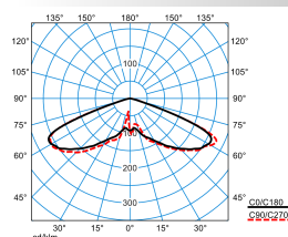
Publisca P1-RB6L/2200-730 3G1S
