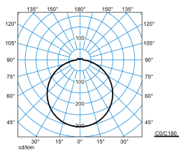
Olisq RWD2 DW 20-830 ET IP54 PC + Olisq RWD2 ZDR 1/2 01
