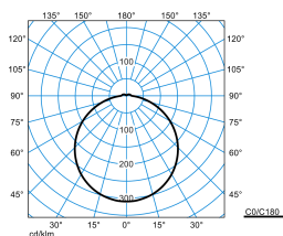
Olisq RWD2 DW 20-830 ET IP54 PC + Olisq RWD2 C 01
