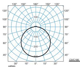
Olisq RWD2 DW 20-830 ET IP54 PC + Olisq RWD2 ZDR 1/2 05
