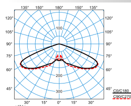
Publisca P2-RB6L-LR/5100-730 6G1S ET (CLO initial value)
