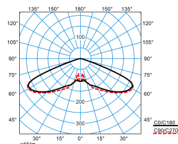
Publisca P2-RB6L-LR/5100-730 6G1S ET (CLO end value)
