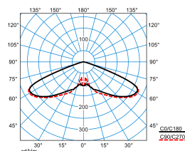
Publisca P2-RB6L-LR/5100-730 6G1S
