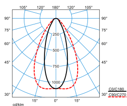
E-Line PRO 78IP50 MironaF T 130-840 ETDD L150 01 ESG Blank (LEO1)
