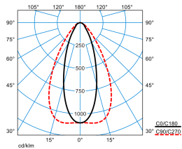
E-Line PRO 78IP50 MironaF T 130-840 ETDD L150 01 ESG 01 IP50 (LEO2)
