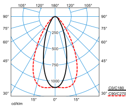
E-Line PRO 78IP50 MironaF T 130-840 ETDD L150 01 ESG Blank IP50 (LEO1)
