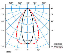
E-Line PRO 78IP50 MironaF T 130-840 ETDD L150 01 ESG 01 (LEO2)
