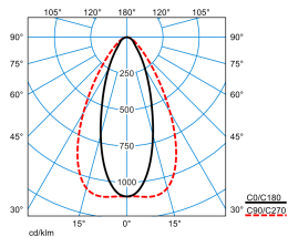
E-Line PRO 78IP50 MironaF T 130-840 ETDD L150 01 ESG 01 IP50 (LEO1)
