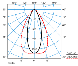
E-Line PRO 78IP50 MironaF T 130-840 ETDD L150 01 ESG Blank (LEO2)
