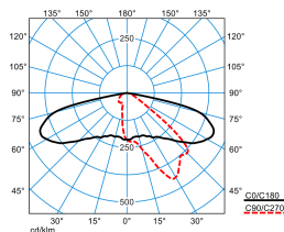
Cuvia60-AB2L8S3-82-740-ET-CAB-26 (CLO end value)
