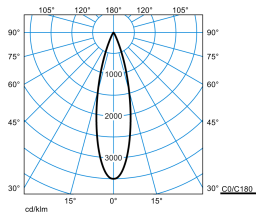
E-Line PRO 78 Lentyp L-MF 40-835 M34 ET 03 Blank
