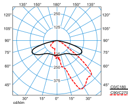
Publisca P1-AB2L-LR/3200-730 4G1S
