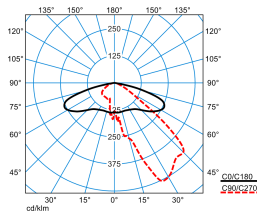
Publisca P1-AB2L-LR/3200-730 4G1S ET (CLO initial value)
