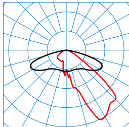
Publisca P1-AB2L-LR/3200-730 4G1S ET (CLO end value) TX300577 ■ C0 - C180 ■ C90 - C270 DIN 5040: A30 UTE: 1,00 G DLOR: 100 % ULOR: 0 % CEN Flux Code: 35 73 97 100 100
