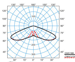
Publisca P1-RB6L-LR/1800-740 2G1S ET (CLO end value)
