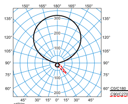
Luceos S-T G3 PAW-IL 300-8TW ETDS 01 (DCW) (LEO1)
