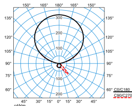
Luceos S-T G3 PAW-IL 300-8TW ETDS 01 (DSU) (LEO2)
