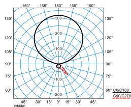
Luceos S-T G3 PAW-IL 300-8TW ETDS 01 (DSU) (LEO1)
