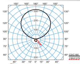
Luceos S-T G3 PAW-IL 300-8TW ETDS 01 (LEO1)
