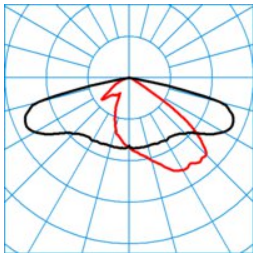
Jovie 70-AB7L-16-135-730-CLO-E
