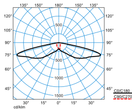
Publisca P3-SB3L-LR/1350-730 2G1 ET (CLO initial value)
