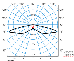
Publisca P3-SB3L-LR/1350-730 2G1 ET (CLO end value)
