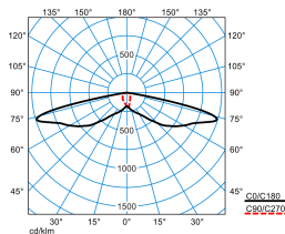
Publisca P3-SB3L-LR/1350-730 2G1
