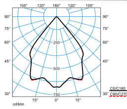
LPCV 3P2 L-W19 05 80-840 K04 ET 05
