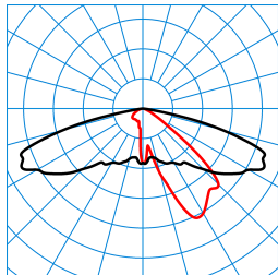
Publisca P1W-AB2L-LRA/4600-740 6G1S ET (CLO end value) TX300911 ■ C0 - C180 ■ C90 - C270 DIN 5040: A30 UTE: 1,00 G DLOR: 100 % ULOR: 0 % CEN Flux Code: 34 72 97 100 100 0 0 0 0
