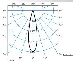
E-Line PRO 78 Lentyp L-SP 40-835 M34 ET 03 03
