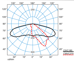
Cuvia60-AB2L12S2-68-7TW-ET-CAB-26 (DWW-CLO initial value)
