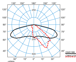
Cuvia60-AB2L12S2-68-7TW-ET-CAB-26 (DCW-CLO end value)
