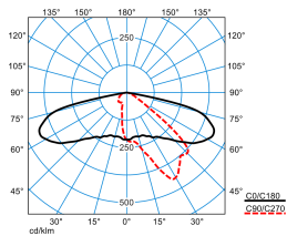
Cuvia60-AB2L12S2-68-7TW-ET-CAB-26 (DWW-CLO end value)
