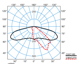
Cuvia60-AB2L12S2-68-7TW-ET-CAB-26 (DSU-CLO end value)
