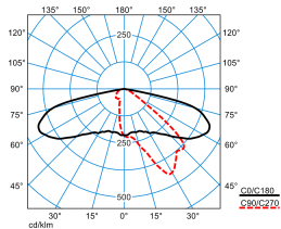
Cuvia60-AB2L12S2-68-7TW-ET-CAB-26 (DSU-CLO initial value)
