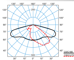
LIQ 70-AB7L/15000-730 14G1S ETDD TX777876
