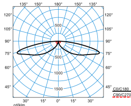
LTX KT-SB3L-LRA/1500-730 2G1 ETDD
