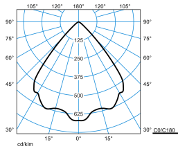
InperlaLP C05 HR22 IP 1800-830 ET 01 TX768981
