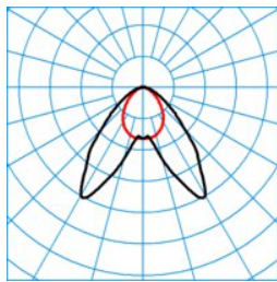
ELINE FL LDAW80 865 L150 1 20 ■ C0 - C180
