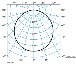
Olisq RWD3 DW 50-8TW ETDD8 IP54 + RWD3 ZDR 1/1 01 (DCW)
