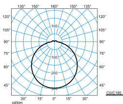
Olisq RWD3 DW 50-8TW ETDD8 IP54 + RWD3 ZDR 1/2 01 (DWW)
