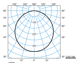
Olisq RWD3 DW 50-8TW ETDD8 IP54 + RWD3 ZDR 1/1 03 (DSU)
