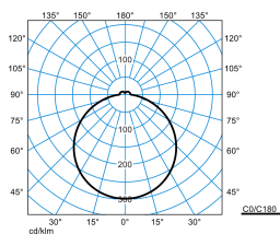
Olisq RWD3 DW 50-8TW ETDD8 IP54 (DSU)
