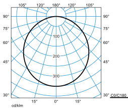
Olisq RWD3 DW 50-8TW ETDD8 IP54 + RWD3 ZVF 03 (DWW)
