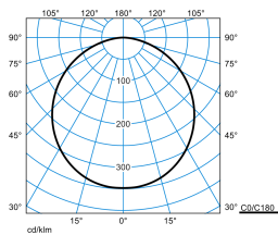
Olisq RWD3 DW 50-8TW ETDD8 IP54 + RWD3 ZDR 1/1 03 (DCW)
