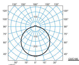
Olisq RWD3 DW 50-8TW ETDD8 IP54 (DSU)
