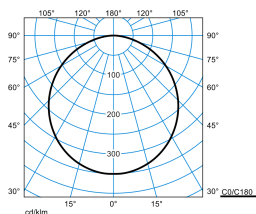
Olisq RWD3 DW 50-8TW ETDD8 IP54 + RWD3 ZVF 03 (DCW)
