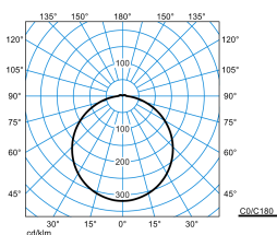
Olisq RWD3 DW 50-8TW ETDD8 IP54 + RWD3 C 01 (DWW)
