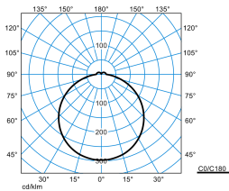
Olisq RWD3 DW 50-8TW ETDD8 IP54 + RWD3 ZDR 1/2 01 (DCW)
