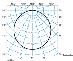
Olisq RWD3 DW 50-8TW ETDD8 IP54 + RWD3 ZVF 05 (DCW)
