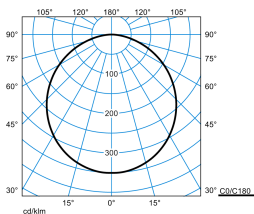
Olisq RWD3 DW 50-8TW ETDD8 IP54 + RWD3 ZVF 01 (DWW)
