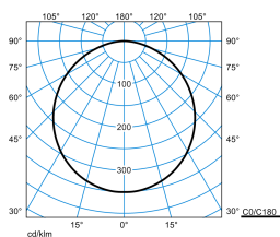
Olisq RWD3 DW 50-8TW ETDD8 IP54 + RWD3 ZVF 01 (DCW)
