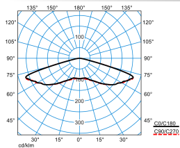
7650 L-SLB 230V Inotec L37 05 (150)
