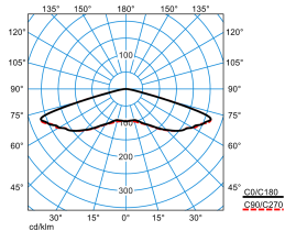
7650 L-SLB 230V Inotec L37 05 (225)
