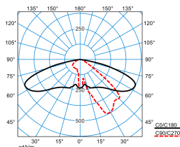
Publisca P1-AB2L/4600-740 6G1S ETDD (CLO initial value) TX300782 DIN 5040: A30 UTE: 1,00 G DLOR: 100 % ULOR: 0 % CEN Flux Code: 35 74 97 100 100
