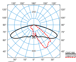
Publisca P1-AB2L/4600-740 6G1S ETDD (CLO end value) TX301293 DIN 5040: A30 UTE: 1,00 G DLOR: 100 % ULOR: 0 % CEN Flux Code: 35 74 97 100 100
