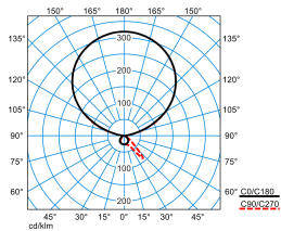
Luceos S-T G3 PAW-IL 300-8TW ETDS 03 (DCW) (LEO2)
