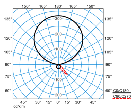
Luceos S-T G3 PAW-IL 300-8TW ETDS 03 (DWW) (LEO1)
