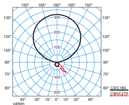
Luceos S-T G3 PAW-IL 300-8TW ETDS 03 (DSU) (LEO2)
