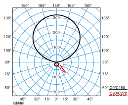
Luceos S-T G3 PAW-IL 300-8TW ETDS 03 (DSU) (LEO1)
