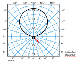
Luceos S-T G3 PAW-IL 300-8TW ETDS 03 (DWW) (LEO2)
