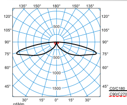
LTX PT-SB3L-LR/1500-740 2G1 ET
