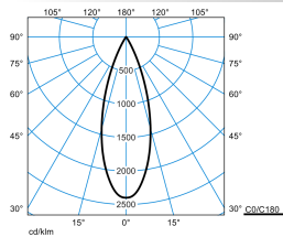
7651 Lentyp L-FL 20-EC M39 ET 03 (150) TX781575
