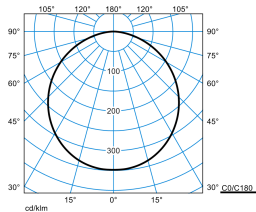
Olisq RWD3 DW 50-830 ETBLE +DMM IP54 + Olisq RWD3 ZDR 1/1 01
