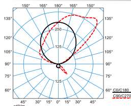
Luceos S G3 PAW-IA 170-940 ETDS KL 05
