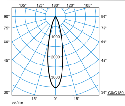
YNSx2LY 7x65 L-MF 05/01 10-930 DD 05 (LEO1)
