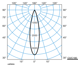
YNSx2LY 7x65 L-MF 05/01 10-930 DD 05 (LEO2)
