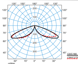
LTX PT-RB6L-LR/2600-730 3G1 ET
