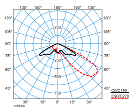
LnPlus 40-AM19L/15000-727 12G1 ETDD (CLO end value)
