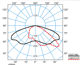
LnPlus 40-AB7L-SLR1/3200-727 4G1 ET (CLO initial value)
