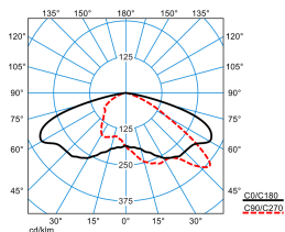
LnPlus 40-AB7L-SLR1/3200-727 4G1 ET (CLO end value)
