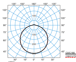
Olisq QWD3 DW 45-840 ET HFS IP54 + Olisq QWD3 ZDR 1/2 03
