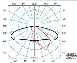
9701SG-AB2L-LR/2600-740 4G2 ET
