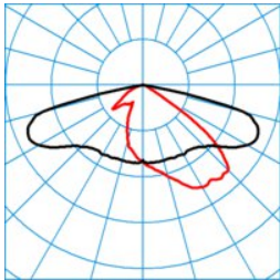
Jovie 70-AB7L-18-165-740-CLO-E
