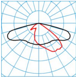
Jovie 70-AB7L-18-165-740-CLO-B
