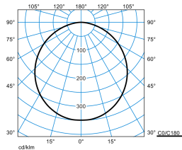
Olisq RWD4 DW 40-830 ET EB3 PC + Olisq RWD4 ZDR 1/1 03
