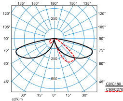
LTX KT-AB2L-SLR/3800-740 4G1 ET
