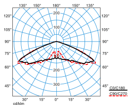
Publisca P1W-RB6L-LR/1500-740 2G1S ET (CLO end value)
