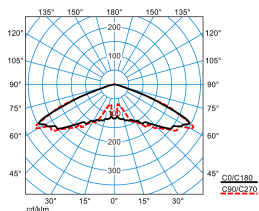
Publisca P1W-RB6L-LR/1500-740 2G1S ET (CLO initial value)
