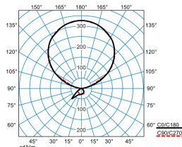
Luceos S-U PAW-IL 300-840 ETDD 05 (LEO2)
