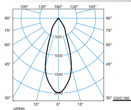
E-Line PRO 78 BV G2 RF-FL 40-EW M48 ET 01 01
