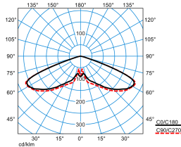
Publisca P2-RB6L-LRA/3200-730 4G1S
