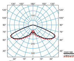
Publisca P2-RB6L-LRA/3200-730 4G1S ET (CLO end value)
