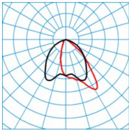
Jovie 70-AM3L-24-240-730-CLO-E
