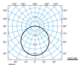
Olisq RWD4 DW 40-830 ETDD IP54 PC + Olisq RWD4 C 01
