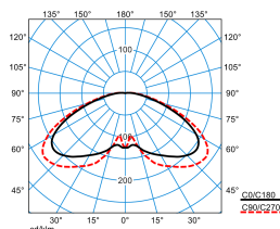
Publisca P1W-RBT-LRA/3800-730 6G1S ET (CLO end value)
