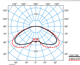
Publisca P1W-RBT-LRA/3800-730 6G1S ET (CLO initial value)
