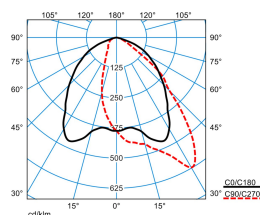
Jovie 70-AM3L-8-82-730-CLO-E
